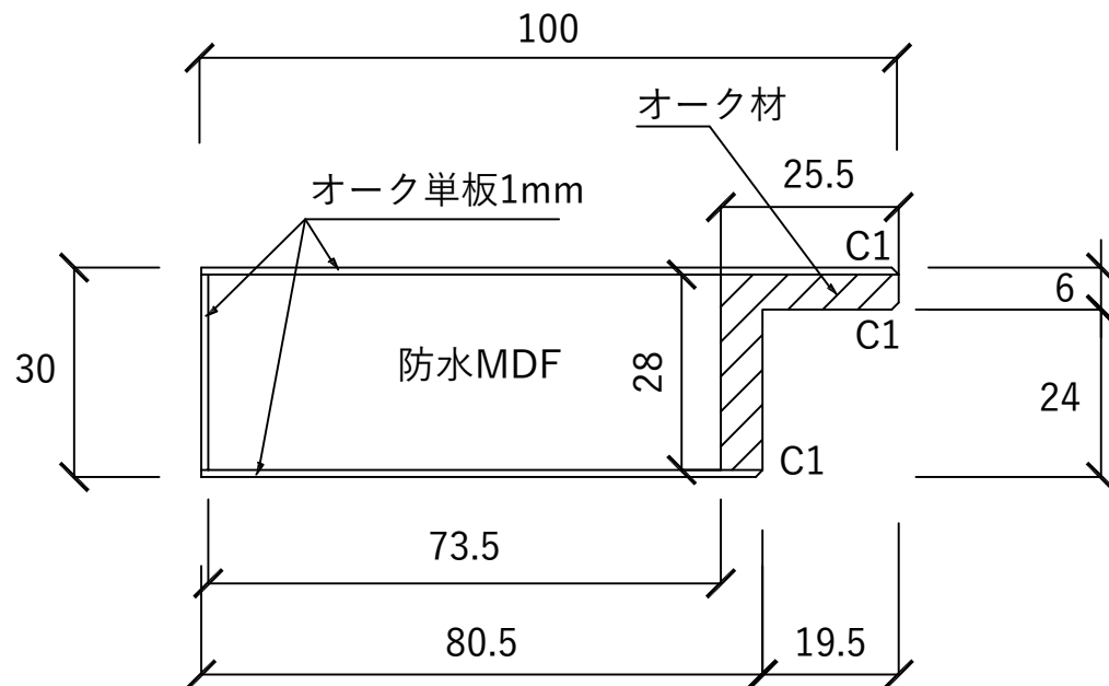
断面図
